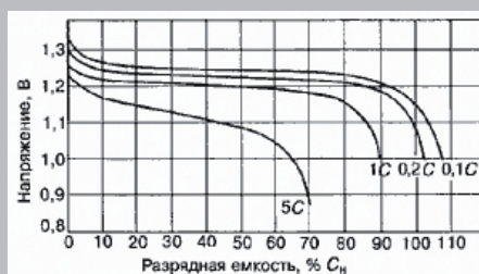
Рис.1. Разрядные характеристики никель-кадмиевого аккумулятора (Ni-Cd) при различных токах разряда
