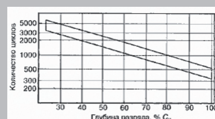
Рис.3. Нарботка герметичных никель-кадмиевых аккумуляторов при разной глубине разряда
