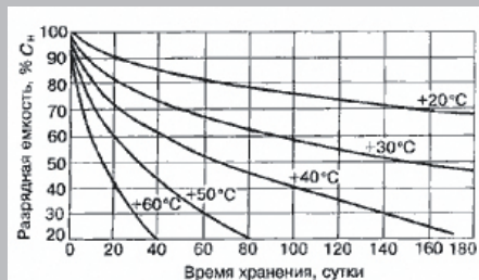
Рис.2. Саморазряд герметичного никель-кадмиевого аккумулятора при различных температурах хранения
